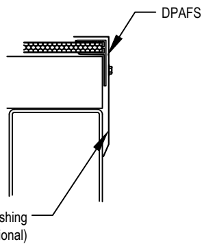
Edge detail
